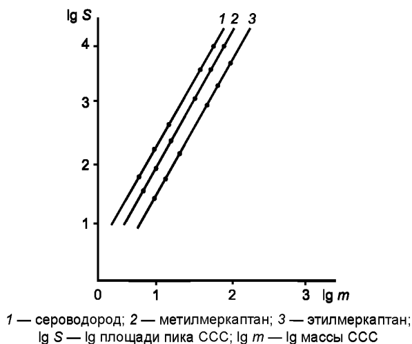
Рисунок 1 — Градуировочный график
